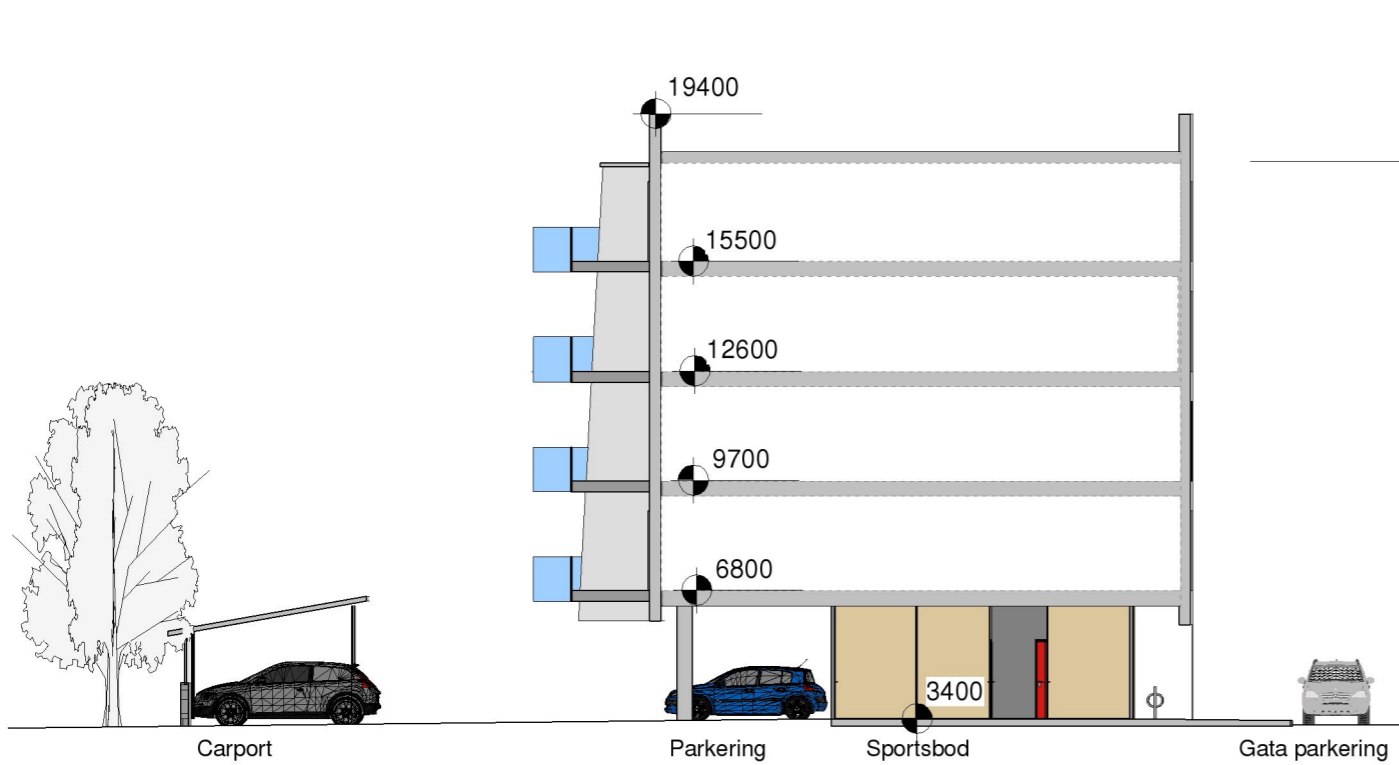
Langsnitt 1 : 200
